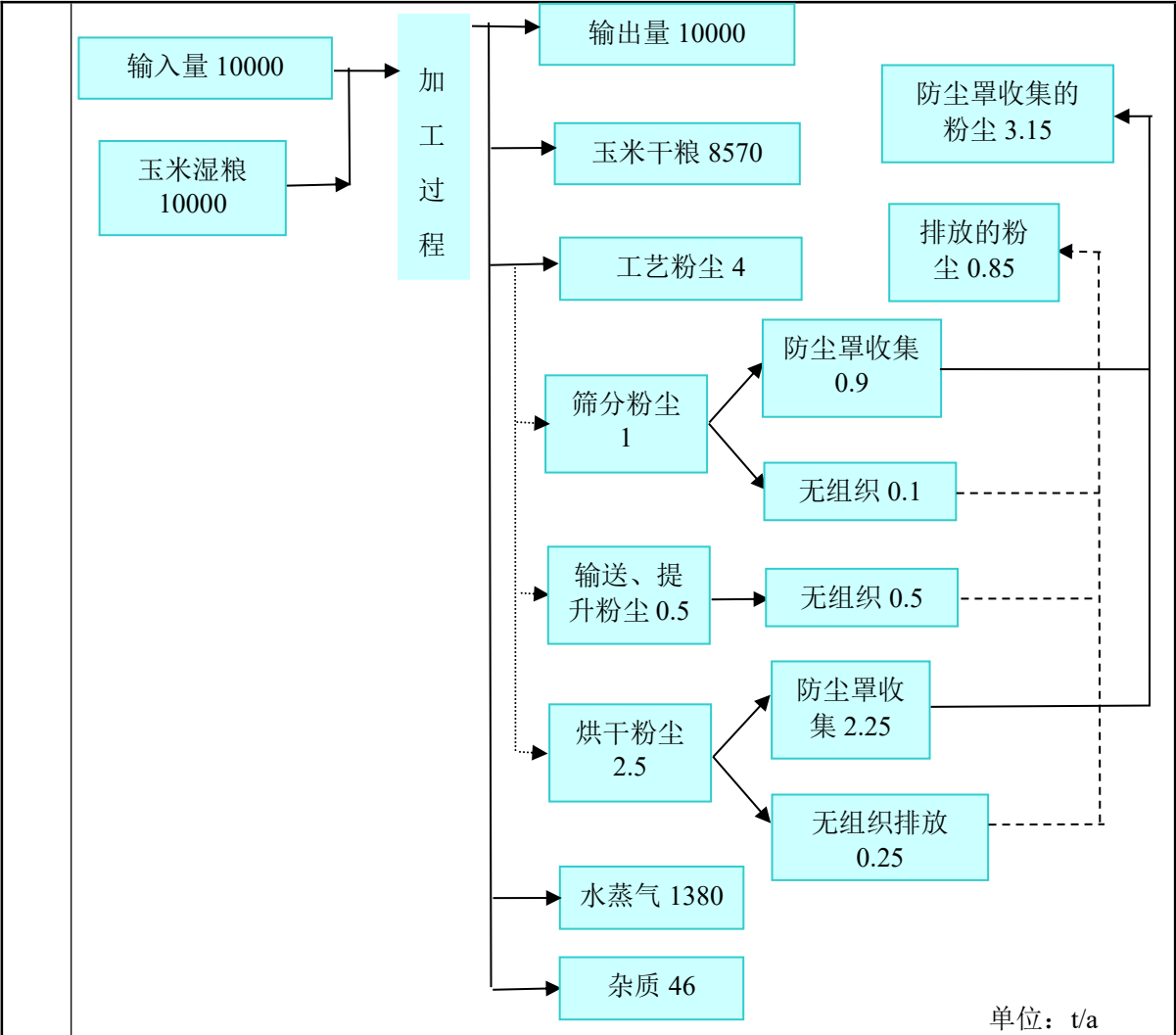
图3 生产物料总平衡图
