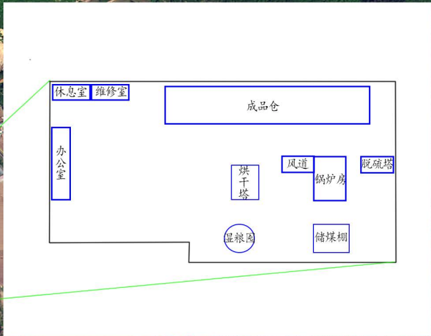
附图4 本项目厂区平面布置图
