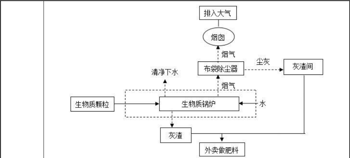
图 2-3 本工程锅炉运行工艺流程及排污工序示意图
