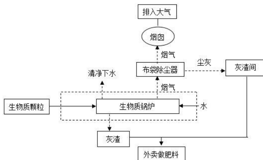
图 2-3 本工程锅炉运行工艺流程及排污工序示意图
