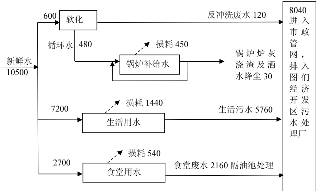
图 2-1 项目给排水平衡图（单位：t/a）
